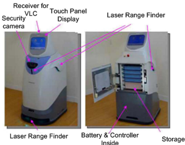
Fig. 6. HOSPI Robot [18].
